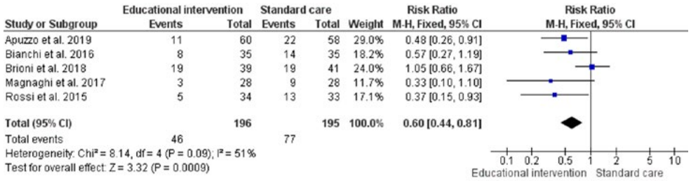
Figure 4: Exemple graphique en forme de forêt
