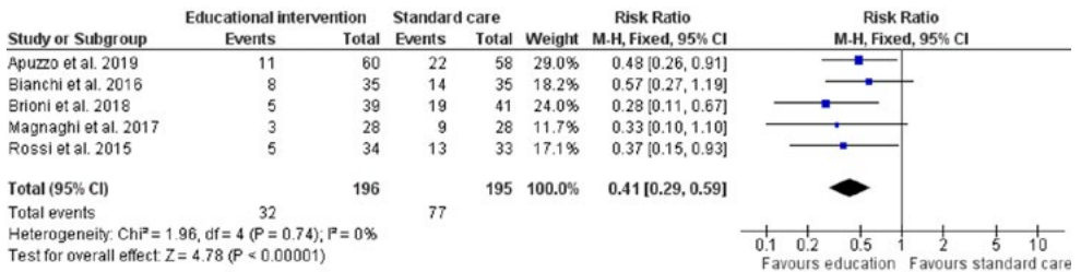
Figure 5: Un graphique en forme de forêt sans hétérogénéité
